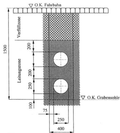
Bild 7. Querschnitt eines mit Boden-Mörtel verfüllten Leitungsgrabens einer Fernwärmeleitung 2 x DN 150 in Übereinanderlage.
