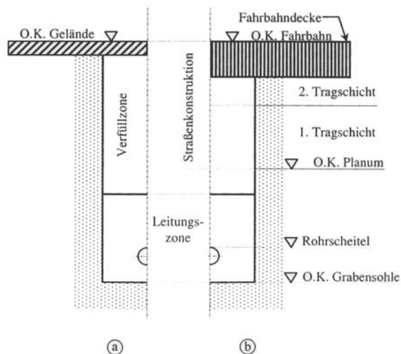
Bild 1. Querschnitt durch einen parallelwandigen unverbauten Leitungsgraben. a) ohne befestigte Oberfläche, b) mit befestigter Oberfläche.
