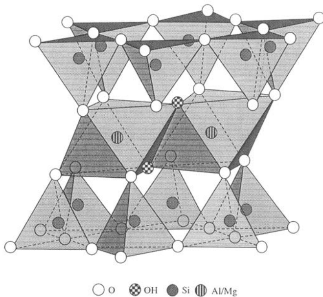
Bild 3. Dreischichtaufbau von Ton nach [13].
