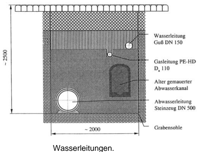
Bild 8. Querschnitt eines mit Boden-Mörtel verfüllten Stufengrabens für die Verlegung von Abwasser-, Gas- und Wasserleitungen.
