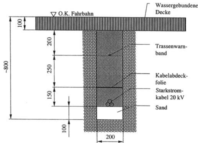
Bild 9. Querschnitt eines mit Boden-Mörtel verfüllten Kabelgrabens, 3 x 20 kV.
