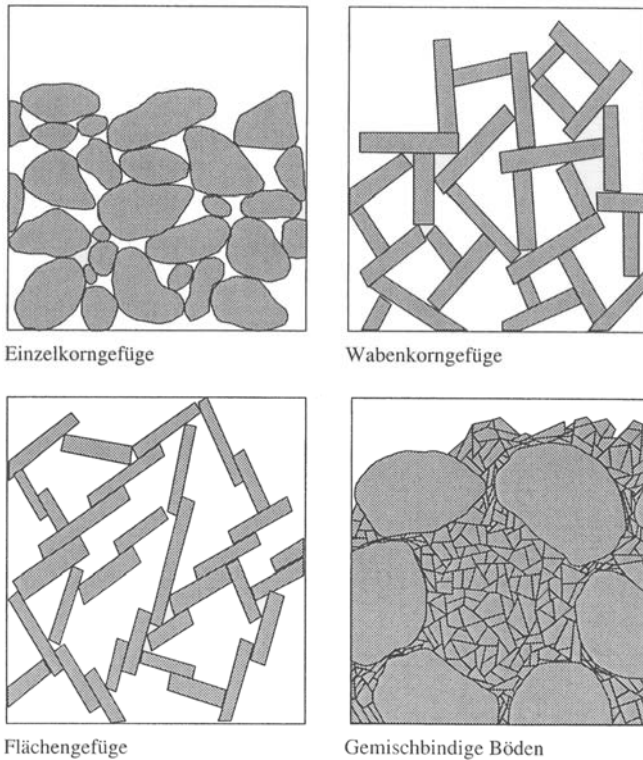
Bild 2. Struktur von Böden nach [11;12].
