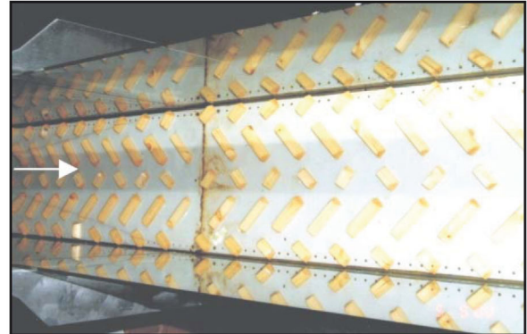
Versetzt und verdreht angeordnete Holzkörper auf ebener Rinnschle (Pfeil Strömungsrichtung)
